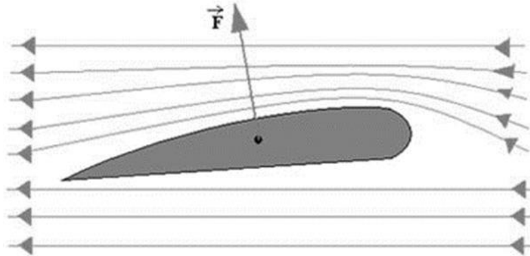
Figura 2: Representação vetorial da força de sustentação em um perfil aerodinâmico
