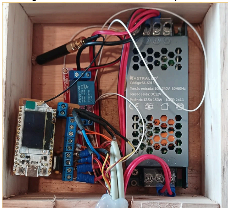
Imagem 2 - Área inferior da caixa com aquecimento
