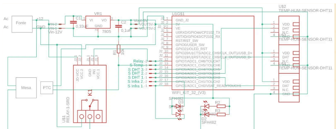
Imagem 5 - Plano elétrico das caixas
