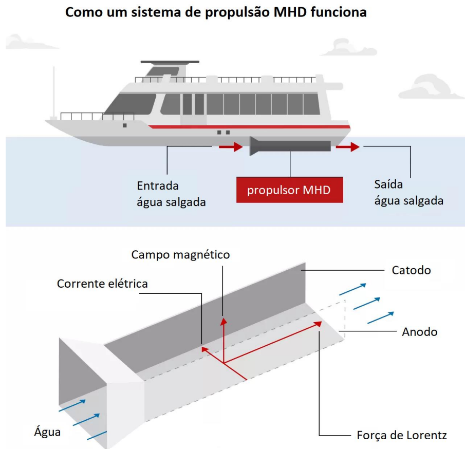
Figura 03 – Como funciona a propulsão MHD.
